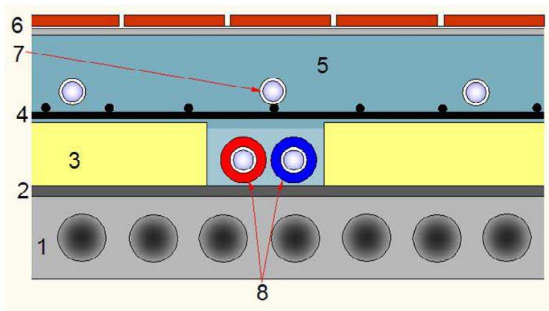
Рис.5.2.р.1 Совместная прокладка труб радиаторного отопления и «теплого пола»
