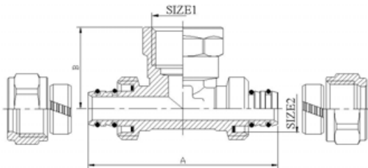
VTm.332 Тройник с переходом на внутреннюю резьбу
