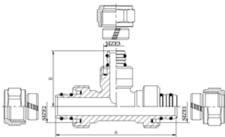
VTm.331 Тройник переходной
