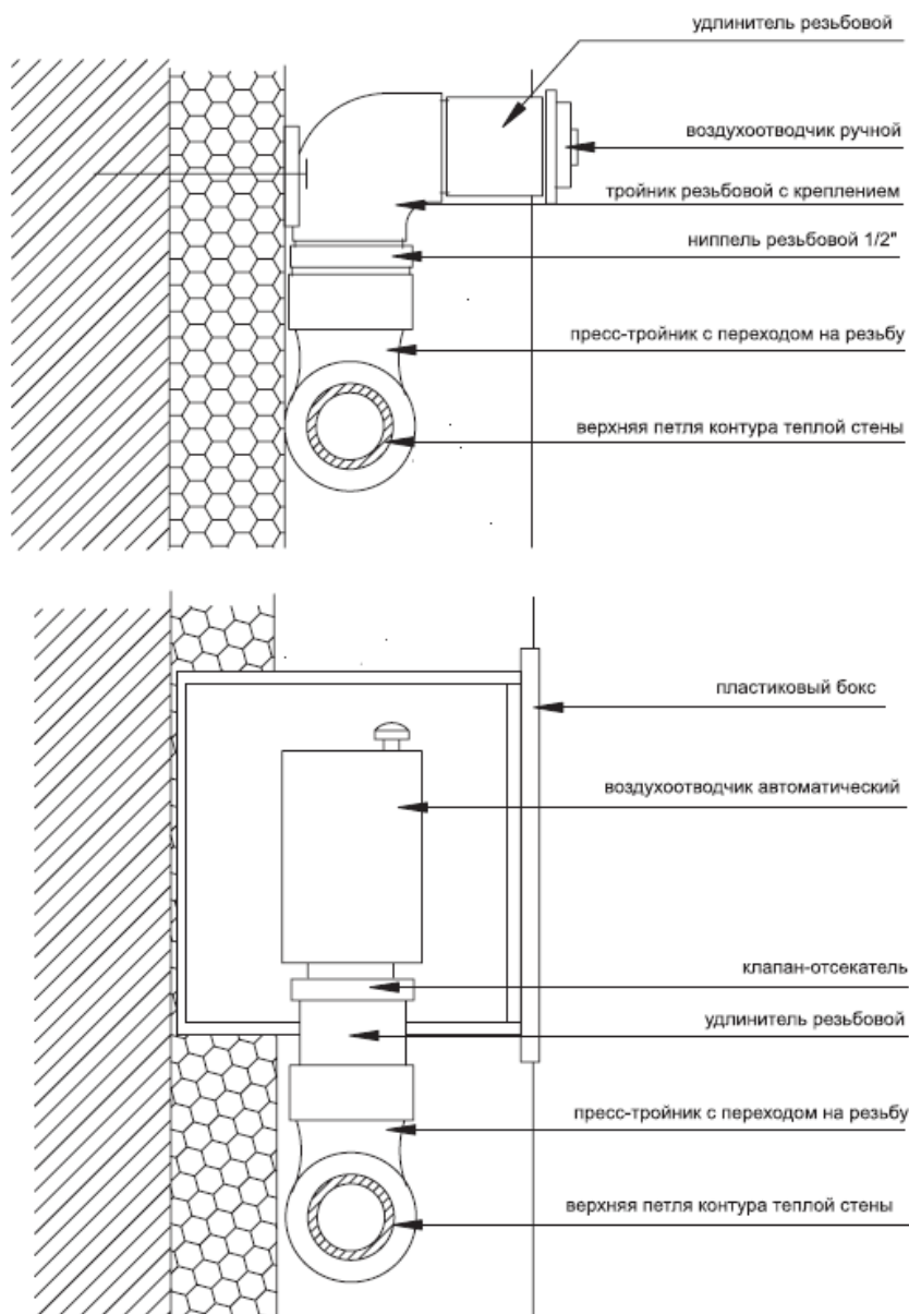
Рис.5.4.р.4 Варианты установки воздухоотводчиков
