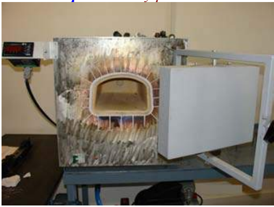
Рис.2.4.3. п.4 Печь муфельная
