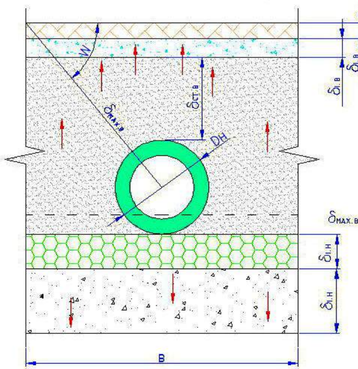
Рис. 6.5.3. р.1 Расчетный элемент теплого пола
