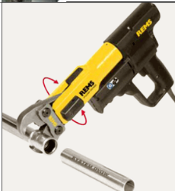
Электрические пресс-клещи
