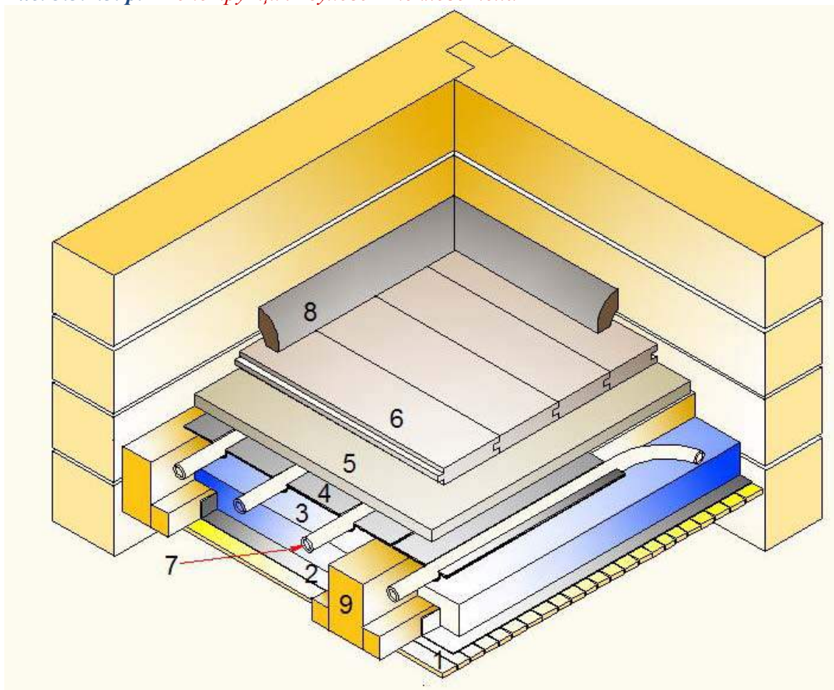
Рис. 5.3.1.3. р.2 Конструкция «сухого» теплого пола
