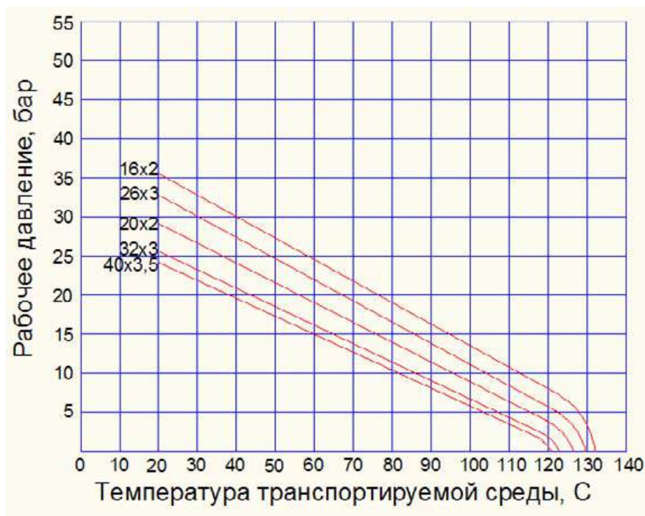
Рис.2.5.5.п.1 График зависимости рабочего давления от температуры транспортируемой среды (из условия срока службы 50 лет)
