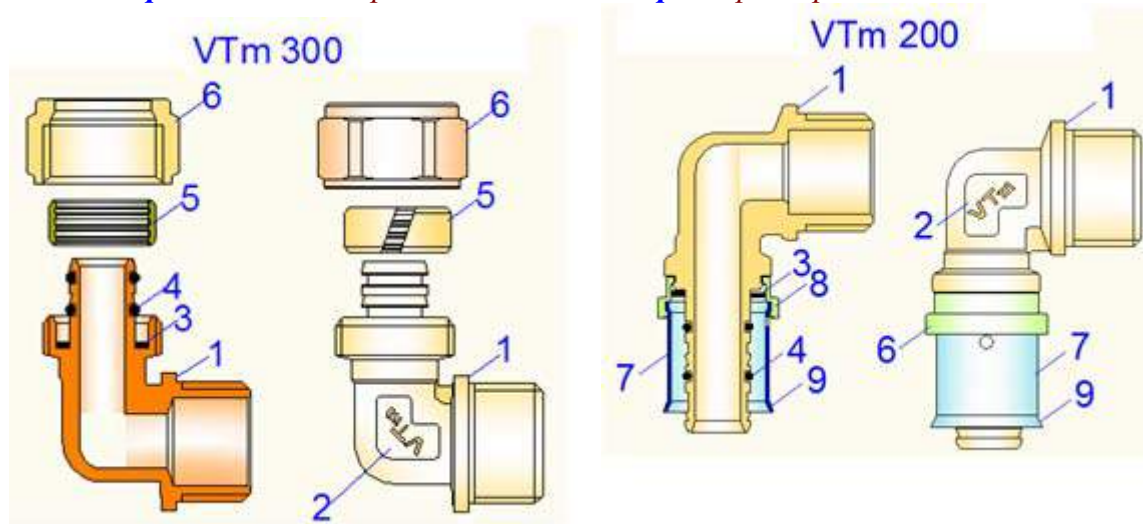
Рис. 3.3.2.р.1. Обжимной фитинг Рис.3.3.2.р.2. Пресс-фитинг
