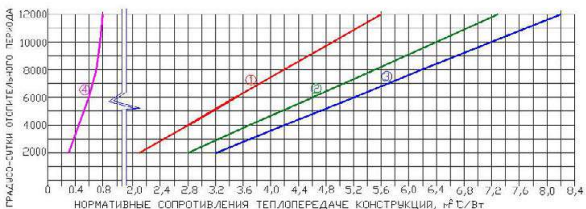
Рис.5.3.1.2.р.2 Требуемые сопротивления теплопередаче ограждающих конструкций (1 – наружные стены; 2 – чердачные перекрытия, перекрытия над подвалами; 3 – покрытия; 4 – окна и балконные двери).
