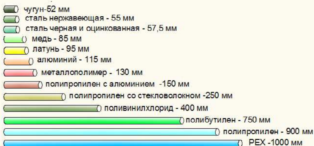
Рис. 2.5.1.р.1 Диаграмма удлинения 100м трубы при повышении температуры на 50 °С
