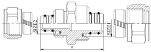
VTm.303 Соединитель переходной
