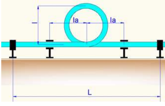
Петлеобразный компенсатор
