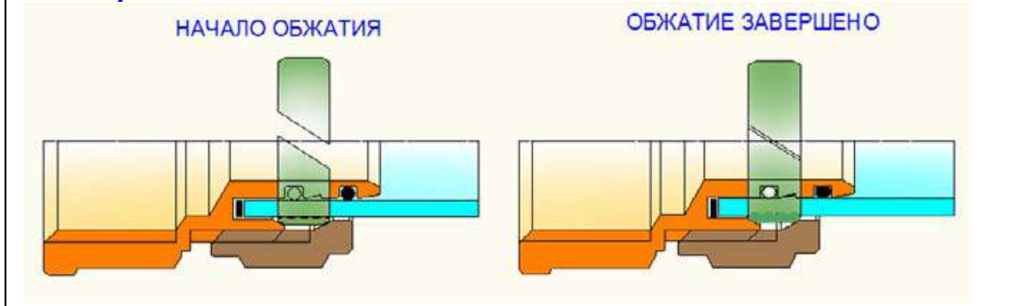
Рис.3.4.р.2. Стадии обжатия МПТ
