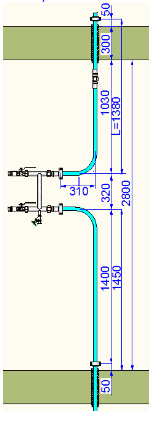
Рис.4.2.4.р.14 Этаже-стояк ГВС
