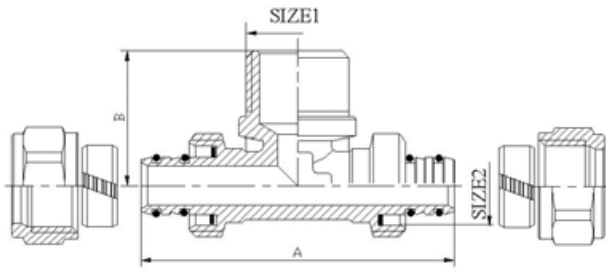
VTm.333 Тройник с переходом на наружную резьбу
