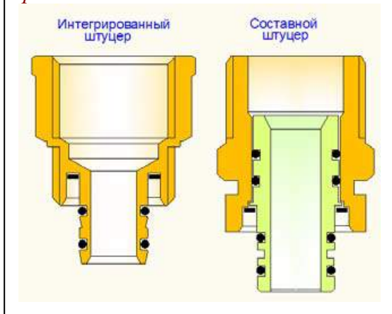
Рис.3.3.5.р.1 Конструкции штуцеров фитингов
