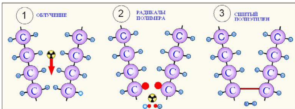
Рис.2.2.р.4 Этапы сшивки полиэтилена по методу С
