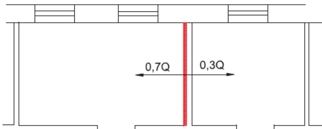
Рис. 5.4.р.2 Отопление двух смежных помещений
