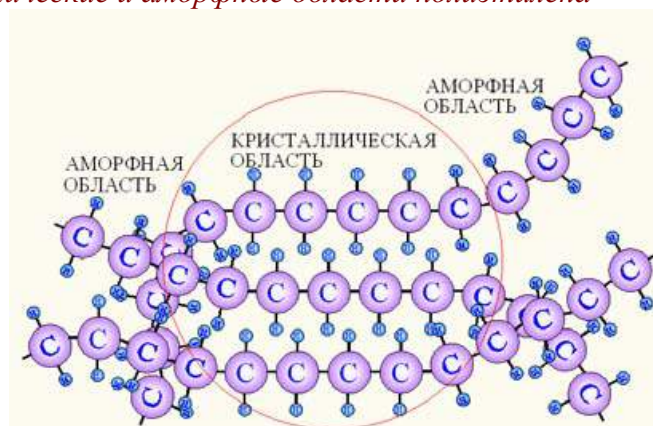
Рис.2.1.р.2 Кристаллические и аморфные области полиэтилена
