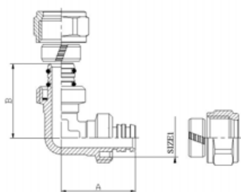
VTm.351 Угольник 90°
