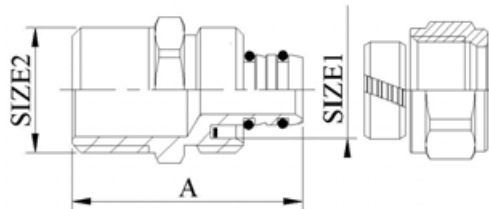
VTm.301 Соединитель с переходом на наружную резьбу
