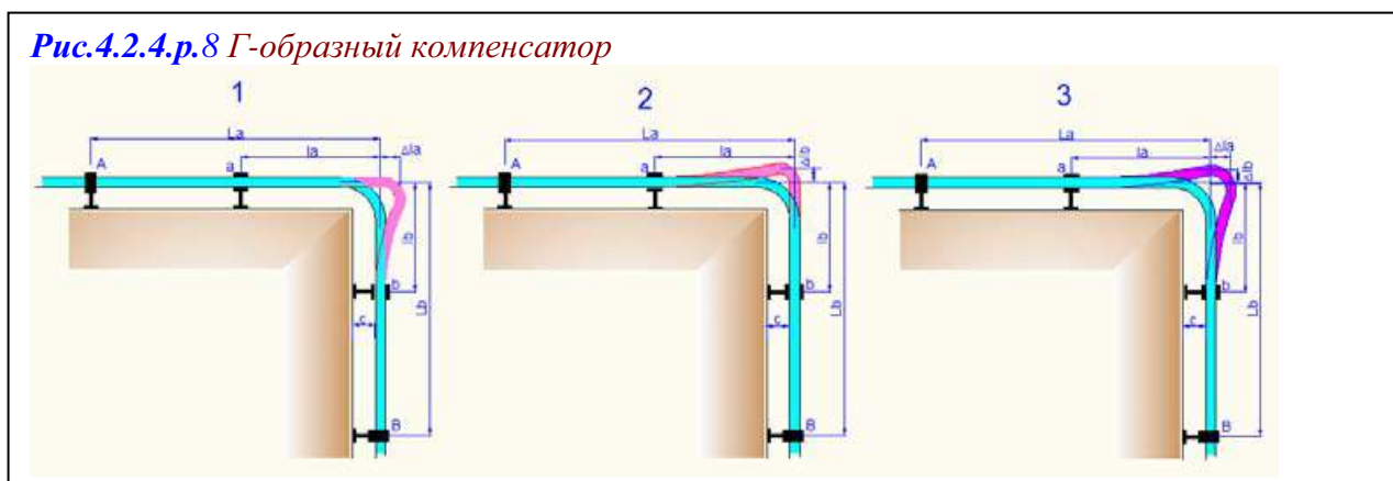
Расчет Г-образного компенсатора (рис.4.2.4.р.8)
