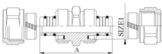
VTm.303 Соединитель
