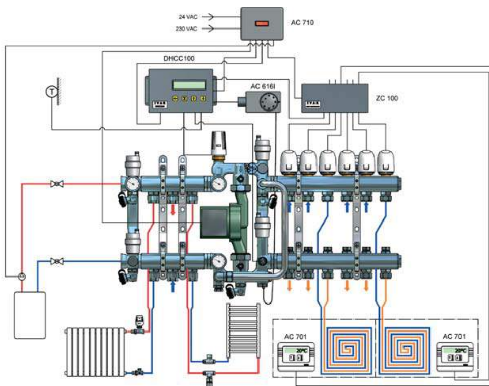
Рис.5.3.1.13 р.3 Комбинированная система отопления с автоматическим управлением
