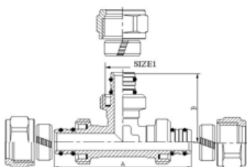
VTm.331 Тройник
