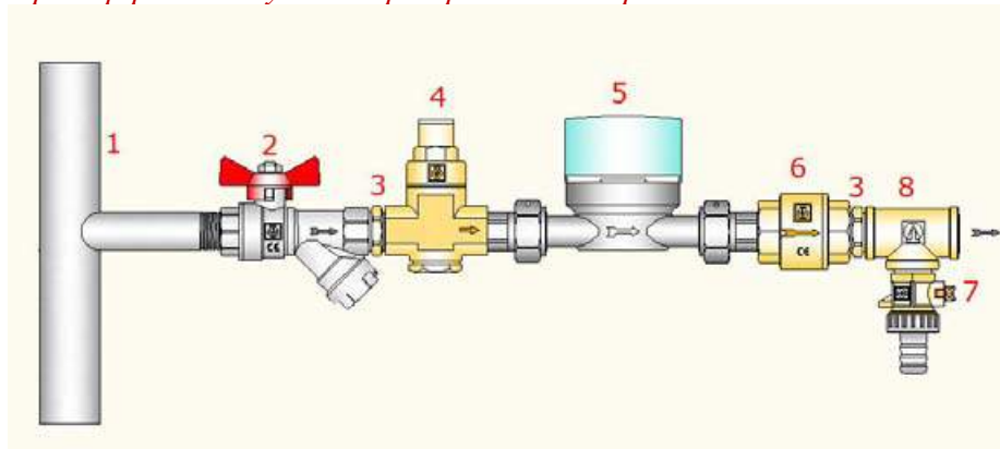
Рис.5.1.р.1 Пример решения узла квартирного водопроводного ввода
