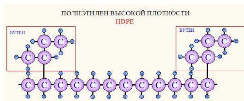
Рис. 2.1.р.3 Химическая структура полиэтилена высокой плотности
