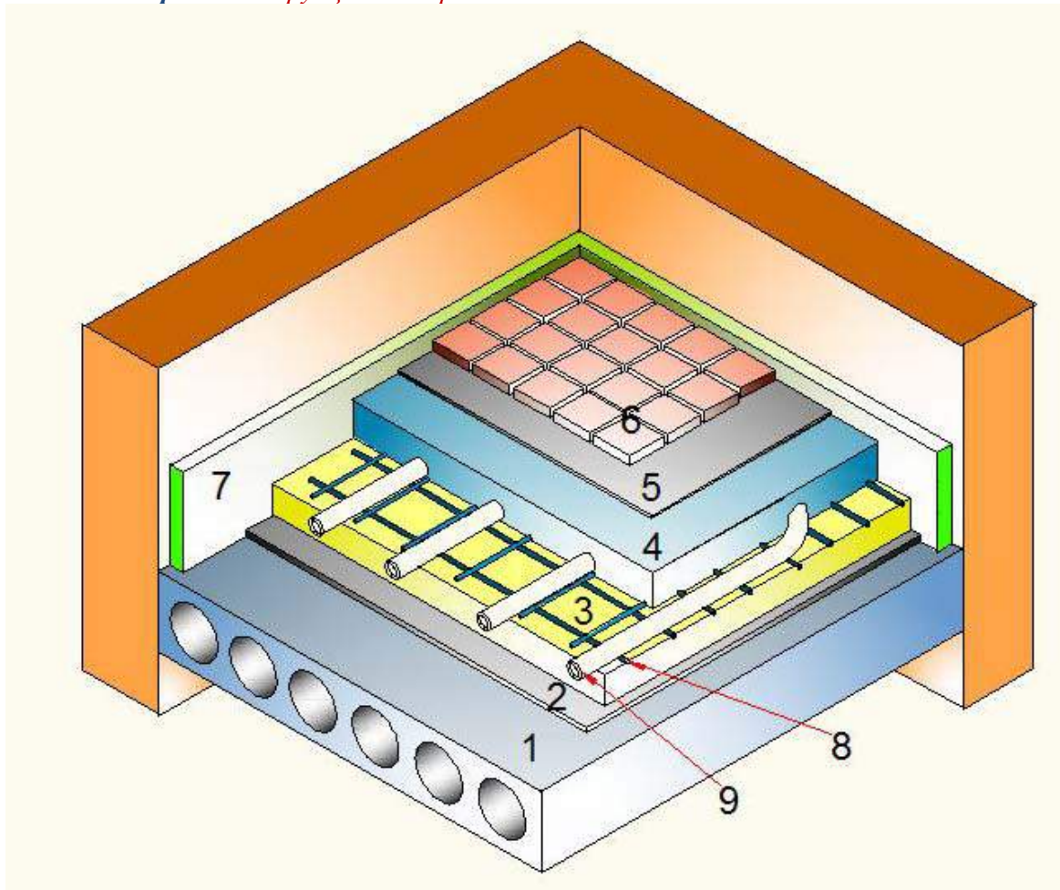
Рис. 5.3.1.3. п.1 Конструкция «мокрого» теплого пола
