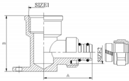
VTm.334 Водорозетка проходная
